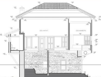
BB KESİTİ
