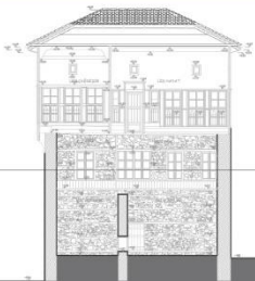
AA KESİTİ
