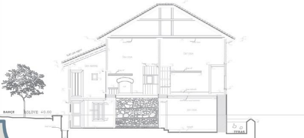
A-A KESİTİ
