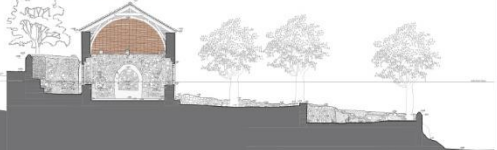
CC KESİTİ
