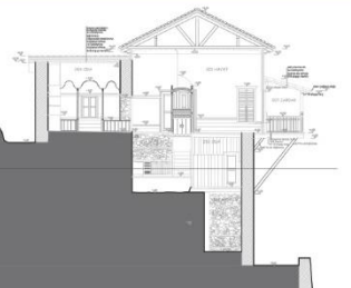
DD KESİTİ
